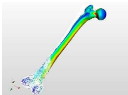
FEM-malli ihmisen reisiluun jännityksistä ja muodonmuutoksista.
