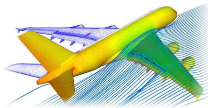
CFD-malli virtaviivoista lentokoneen siiven ympärillä
