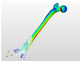
FEM-malli ihmisen reisiluun jännityksistä ja muodonmuutoksista.
